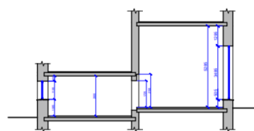
РАЗРЕЗ A-A
