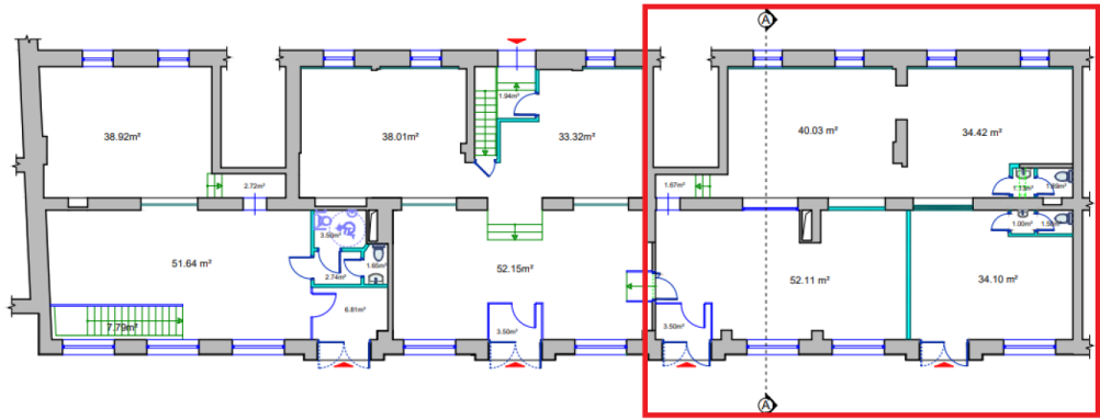
ПЛАН ПОДВАЛА
