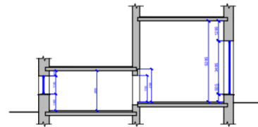
РАЗРЕЗ A-A
