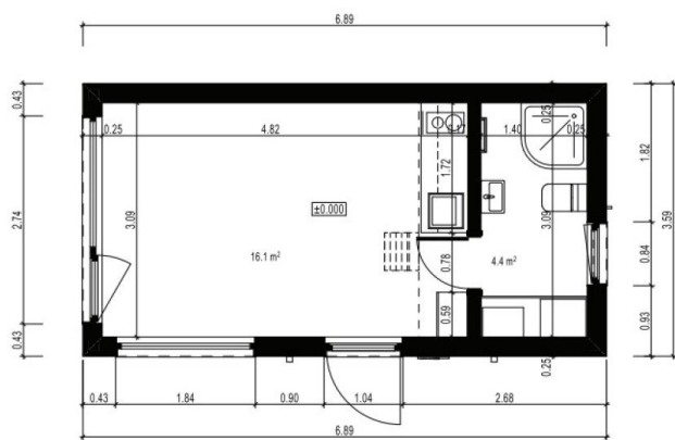
1. STĀVA PLĀNS
