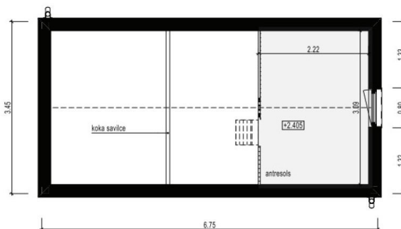
ANTRESOLA PLĀNS
