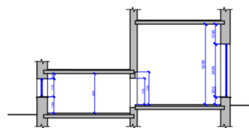
РАЗРЕЗ A-A
